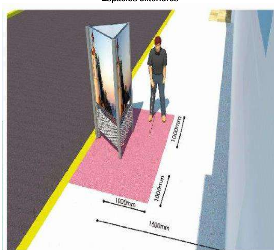
FIGURA A.3 Espacios exteriores
