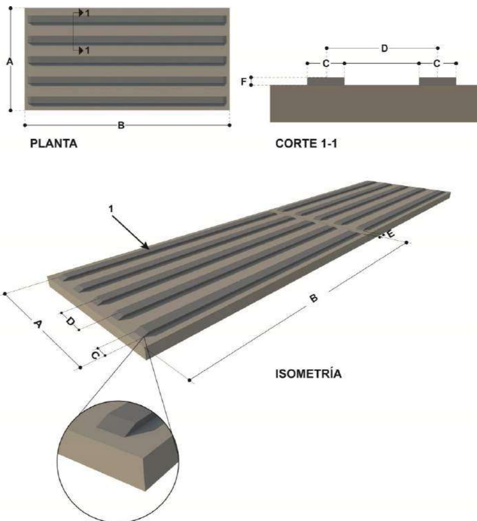
FIGURA 3. Ejemplo ilustrativo. Patrón de alto relieve rectangular segmentado. Dimensiones
