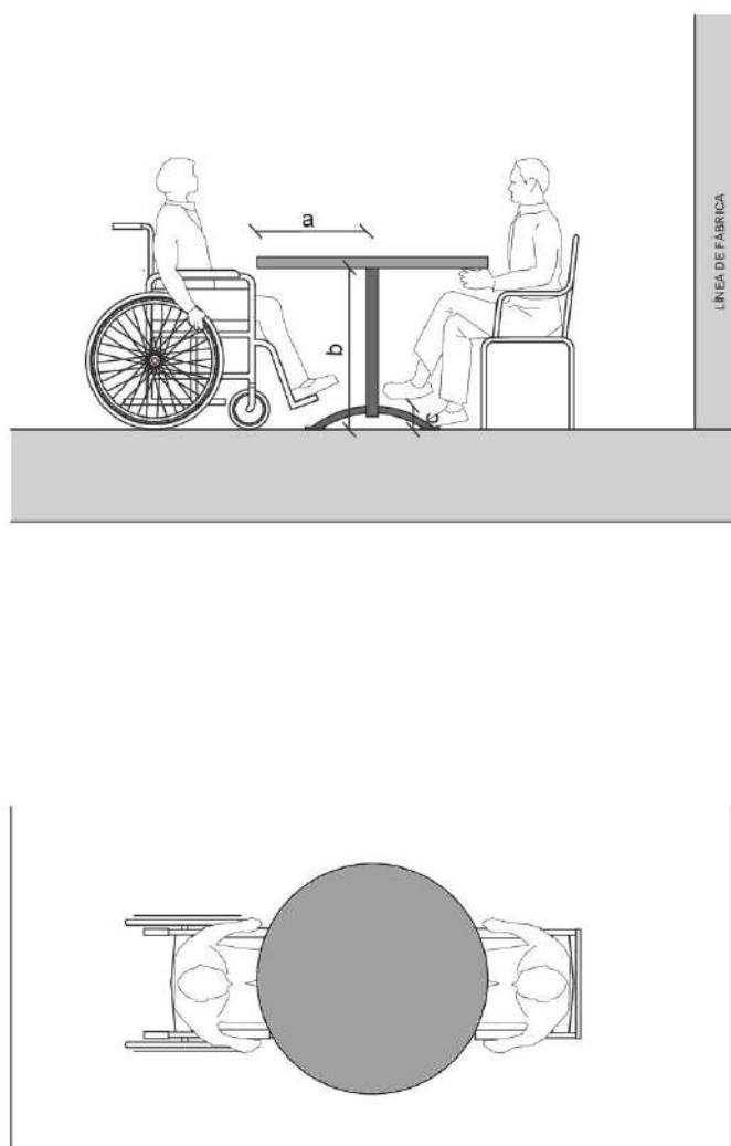
FIGURA 9. Mesas
