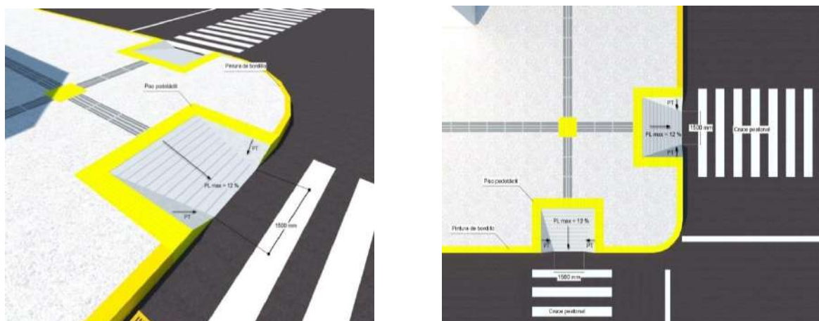
FIGURA 2. Vado de tres planos inclinados
