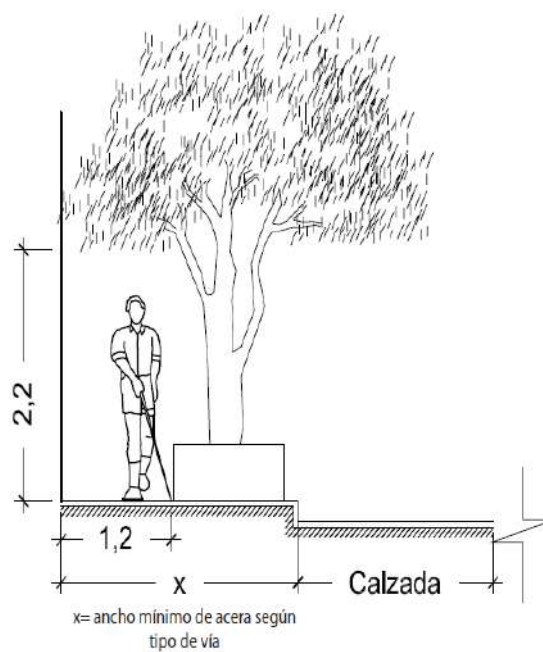
ELEVACIÓN
