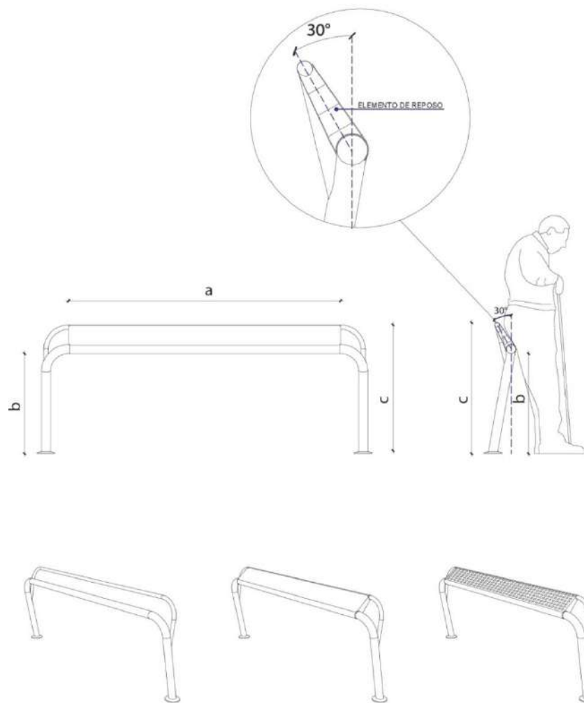
FIGURA 8. Apoyo Isquiático
