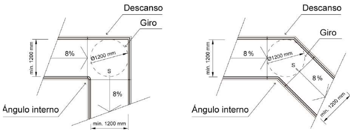
FIGURA 4. Especificación de los literales b) y c)
