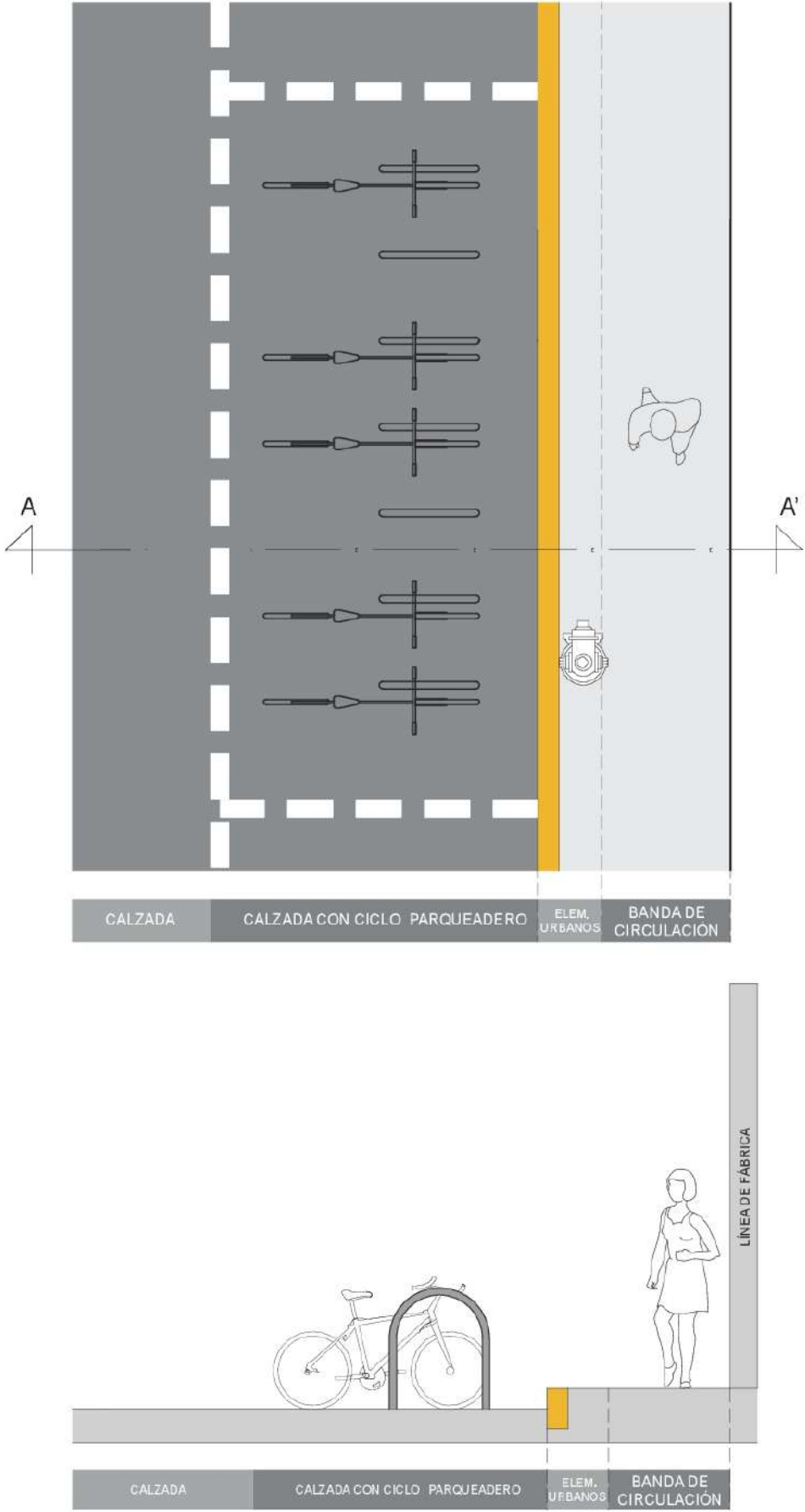
FIGURA 16. Ejemplos de Ciclo Parqueaderos
