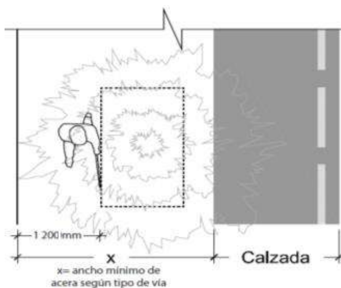
PLANTA
