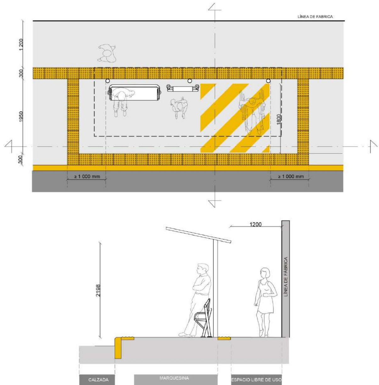
FIGURA 6. Marquesina Tipo
