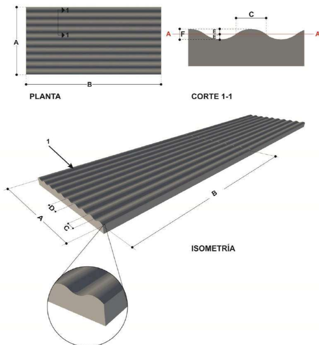
FIGURA 9. Ejemplo ilustrativo. Patrón de alto relieve sinusoidal. Dimensiones.
