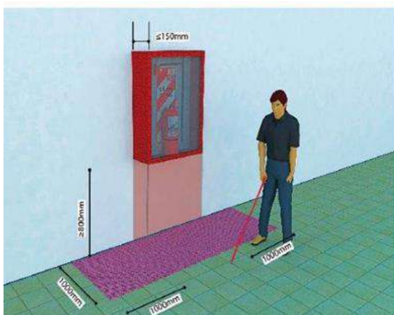
FIGURA A.3 Espacios exteriores
