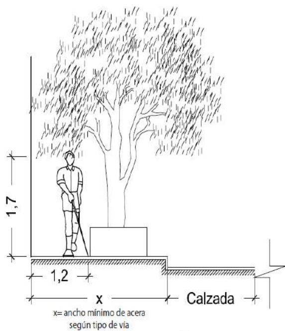
ELEVACIÓN
