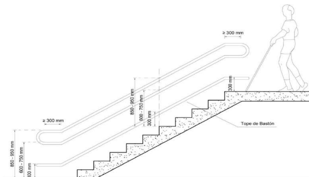
FIGURA 2. Dimensiones para huellas, contrahuellas y altura de pasamanos en escaleras
