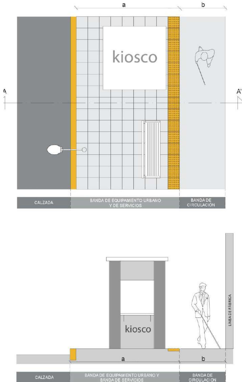
FIGURA 3. Banda de Servicios
