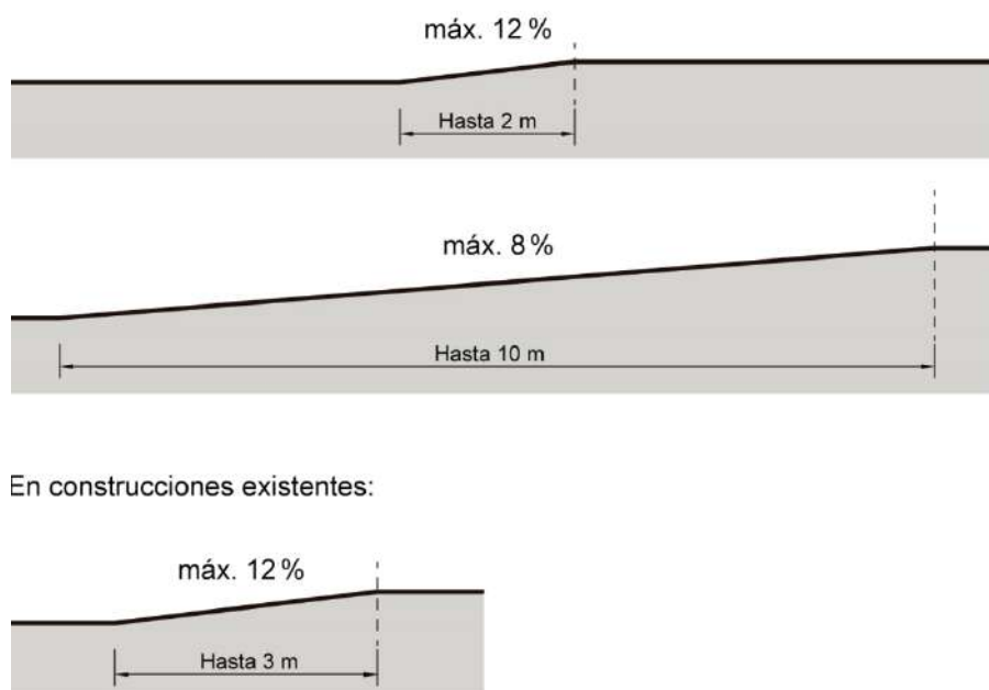
FIGURA 1. Pendientes longitudinales
